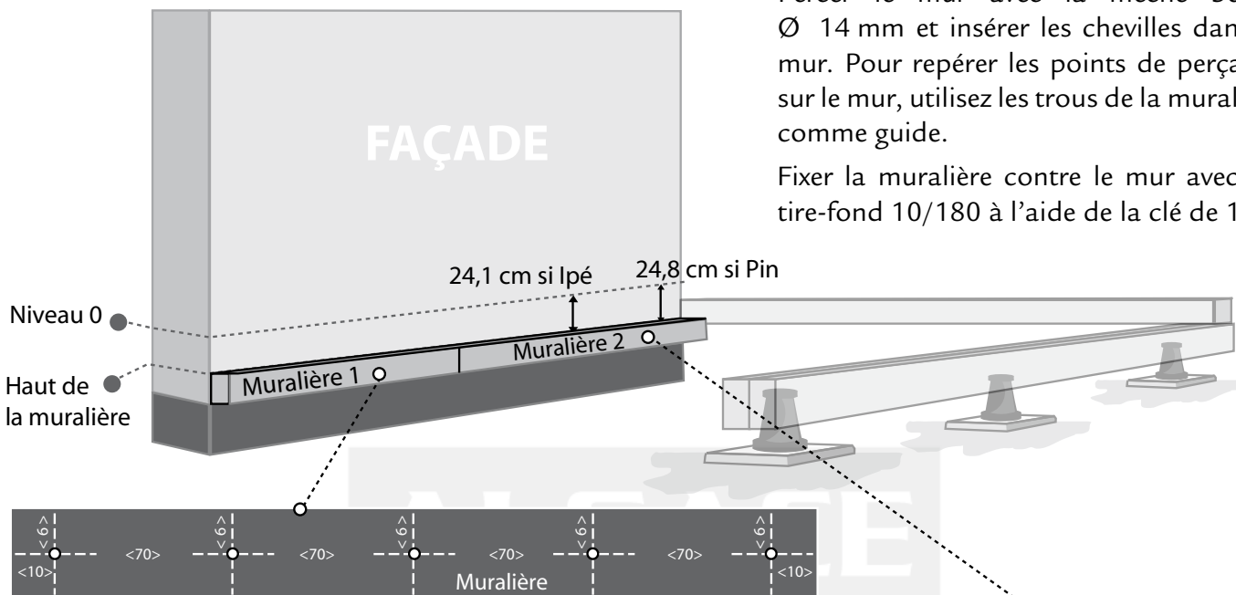
Schéma de perçage muralière 1 (valeur en cm)
